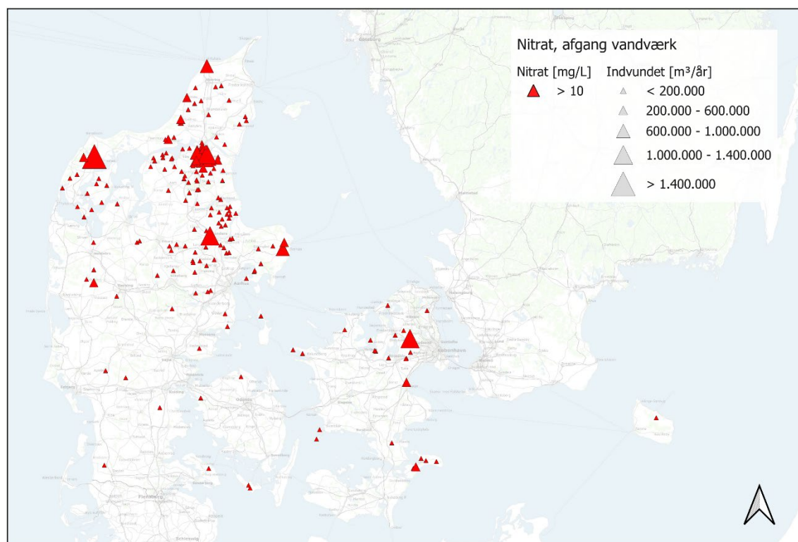
Figur 6 Vandforsyningsanlæg der ikke vil kunne overholde en kravværdi på 10 mg/l.
