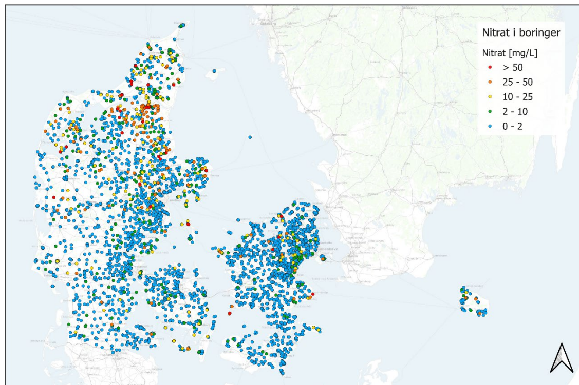
Figur 2 Nitratindhold i almene vandværkers boringer
