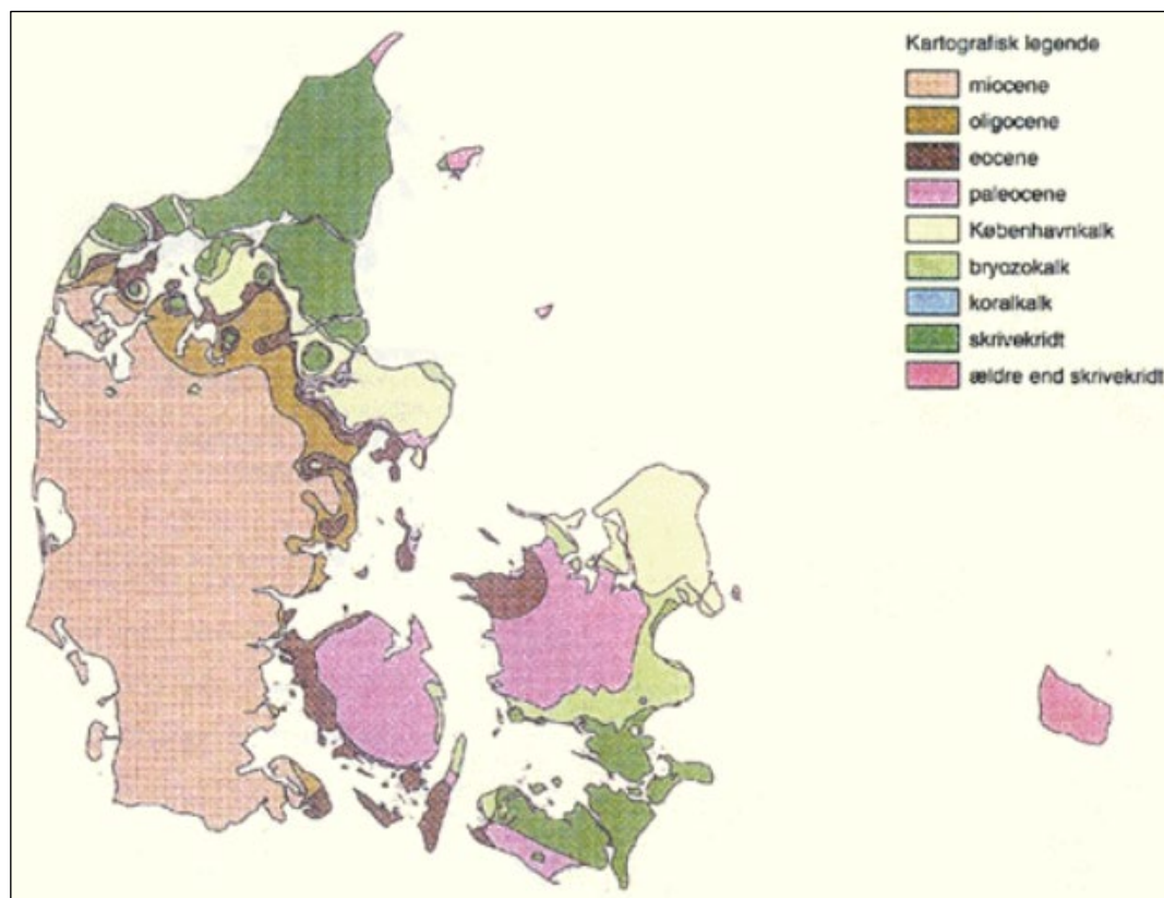
Figur 9 Prækvartær overfladen i DK's undergrund. Kilde GEUS.
